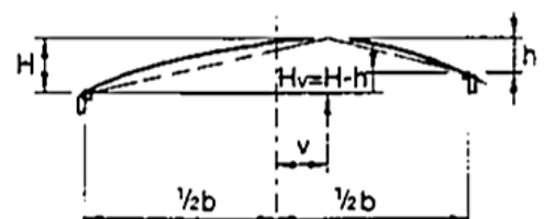
fig. 3.2: Gew. tonrond profiel met verplaatste kruin
